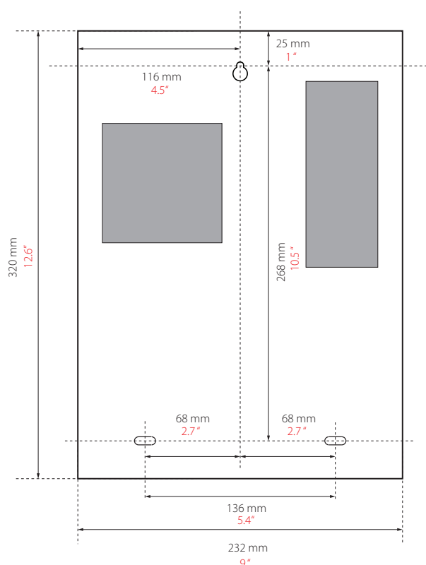
2A 12V gelijkstroomspanning - metalen behuizing 857-693-NL
